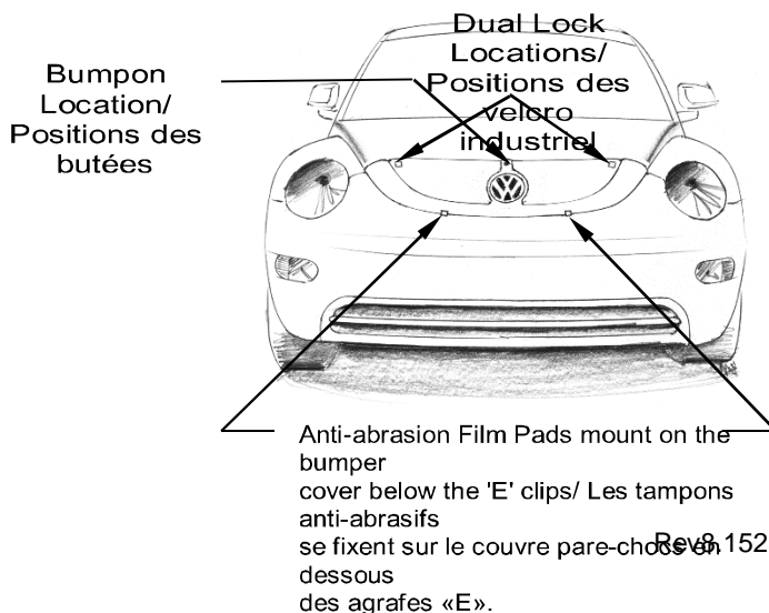
Illustration #2: BUMPONS LOCATION/ Emplacement des butées
